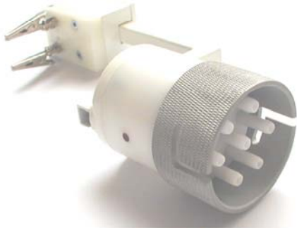
Beispielmessfassung für CCFL-Sockel, U-Form
